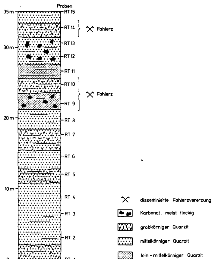
Abb. 4: Profil durch die „Verzerten Quarzite“ im Ramblestobel (1730 m Sh).
